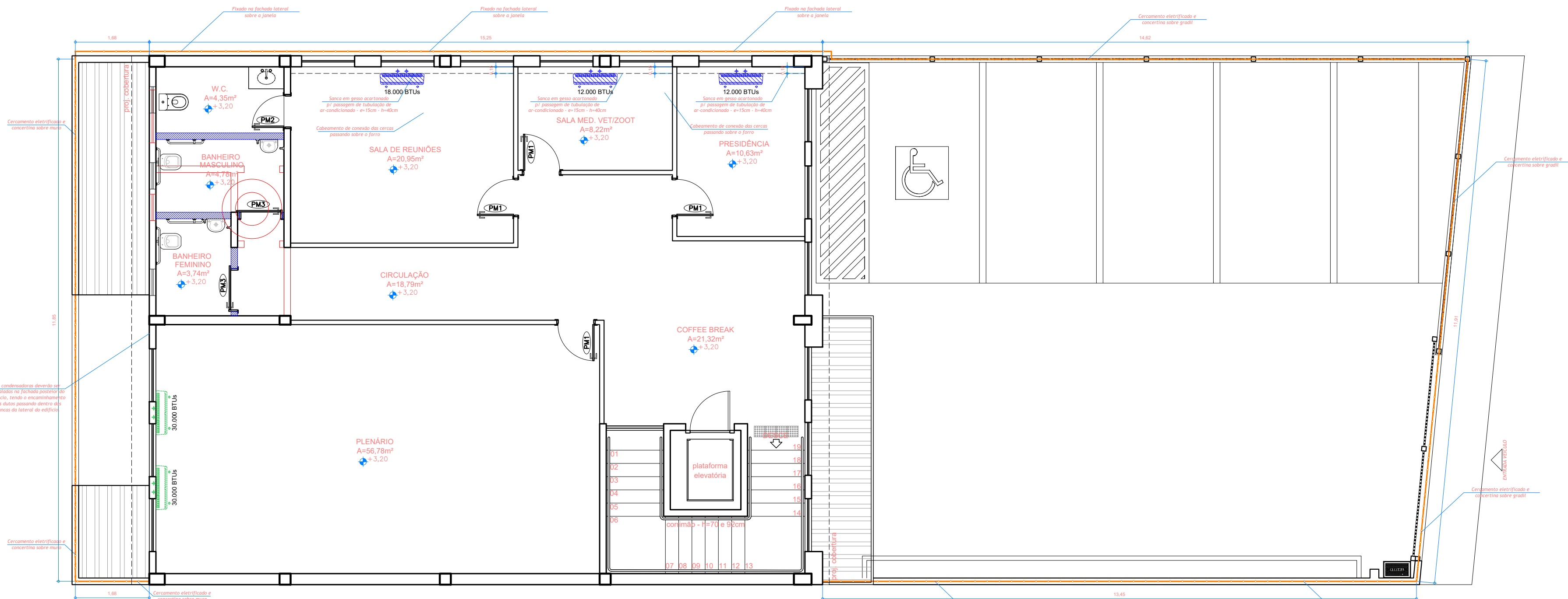
PLANTA-BAIXA PAV. SUPERIOR - CERCAMENTO ELETRIFICADO E CONCERTINA esc.: 1/75
