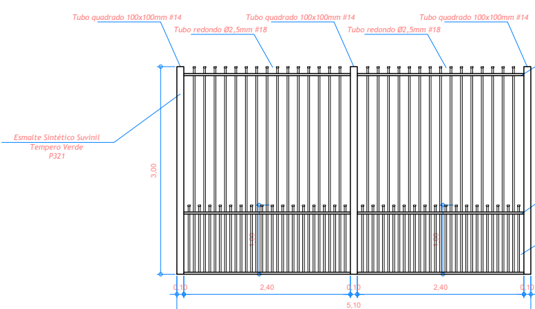
VISTA PORTÃO esc.: 1/75
