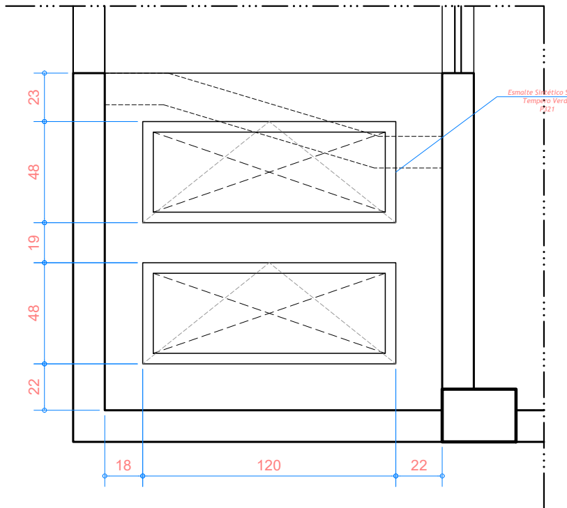
PLANTA-BAIXA TAMPAS esc.: 1/25
