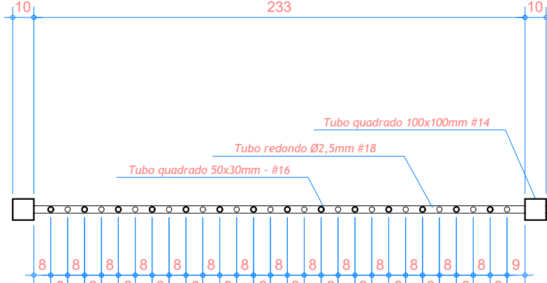
DETALHE ESPAÇAMENTO esc.: 1/25
