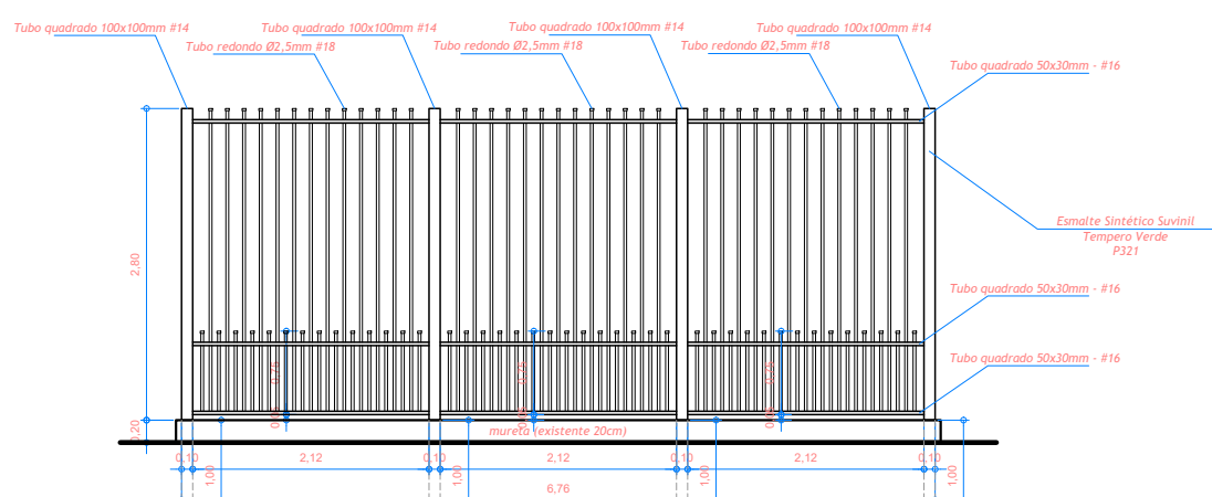
VISTA GRADIL FRONTAL esc.: 1/75
