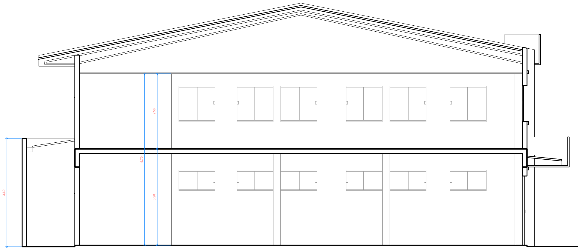
CORTE esc.: 1/75
