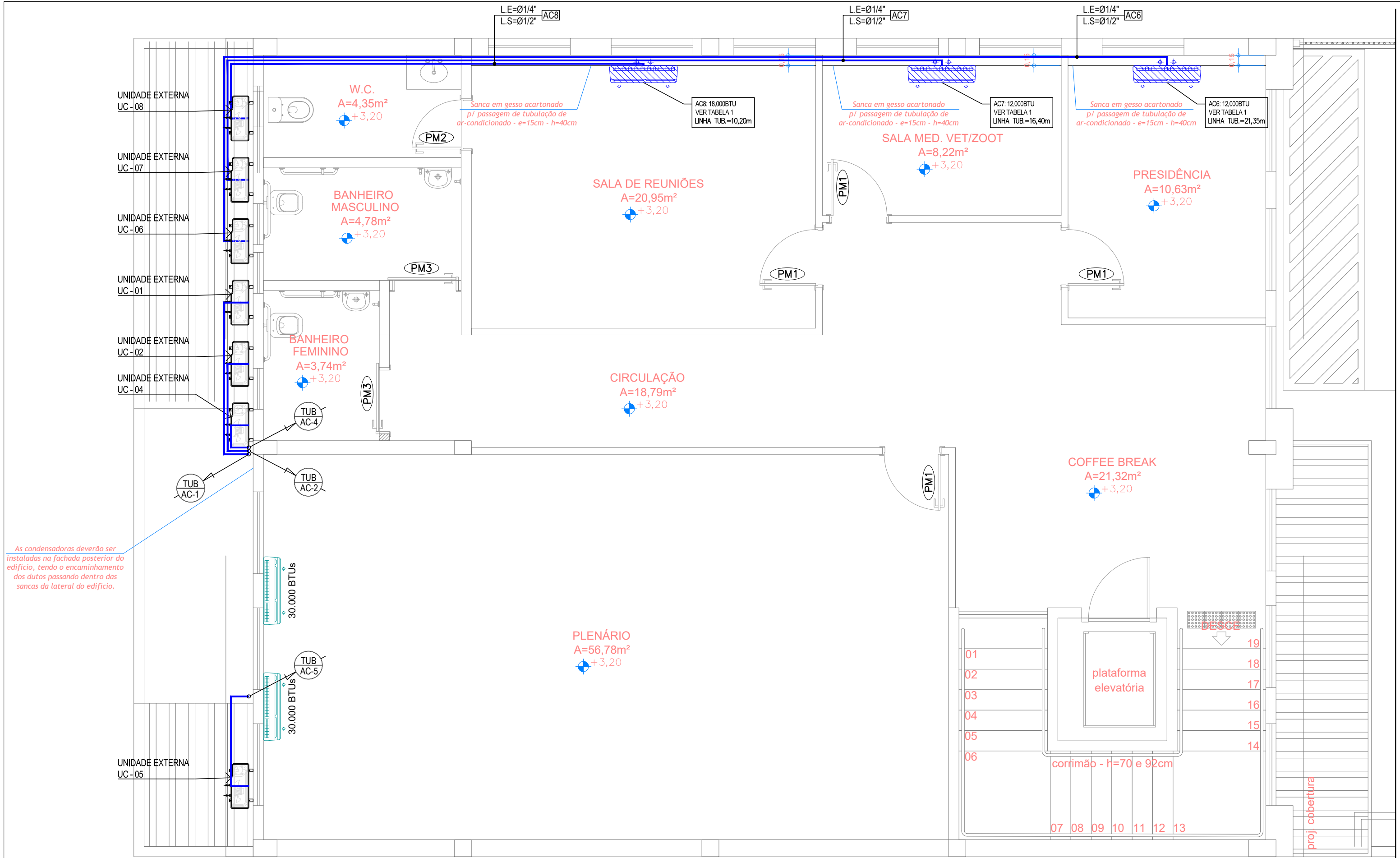
PLANTA-BAIXA PAV. SUPERIOR esc.: 1/75
